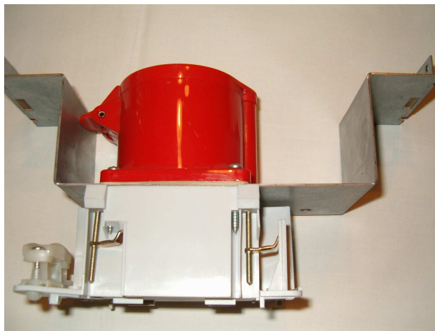
Blacha pod gniazdo CEE, nr katalog. 881 951 010 .
